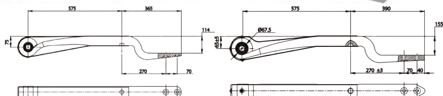
2 PARABOLIC Z SPRING ПОЛУРЕССОРА ПОДВЕСКИ ПРИЦЕПА
