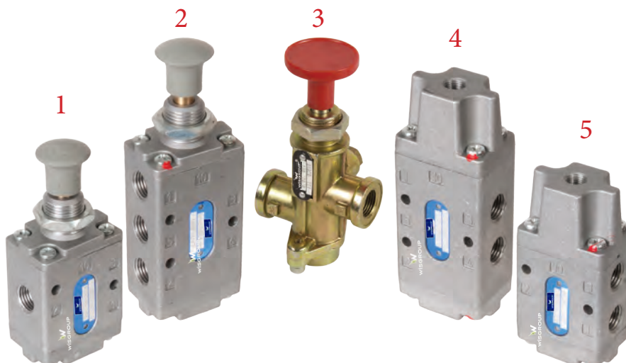
LIFT AXLE CONTROL VALVE РЕГУЛИРУЮЩИЙ КЛАПАН ПОДЪЕМНОЙ ОСИ
