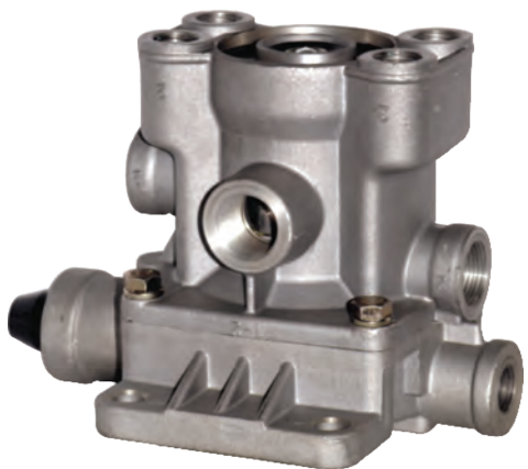
TRAILER BRAKE VALVE ТОРМОЗНОЙ КЛАПАН ПРИЦЕПА
