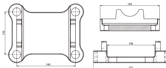
SPRING PAD 100MM W/SHOCK ABSORBER PIN ПРУЖИННАЯ ПОДКЛАДКА/ШТЫРЬ АМОРТИЗАТОРА
