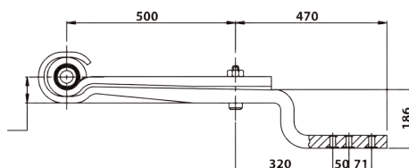
1 PARABOLIC Z SPRING ПОЛУРЕССОРА ПОДВЕСКИ ПРИЦЕПА
