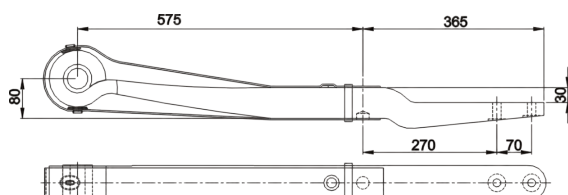
3 PARABOLIC FLAT SPRING ПЛОСКАЯ ПОЛУРЕССОРА
