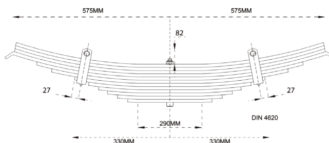
6 LEAF SPRING ЛИСТОВАЯ РЕССОРА
