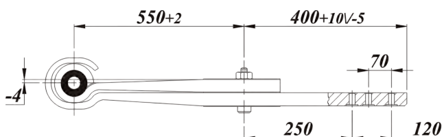
5 PARABOLIC FLAT SPRING ПЛОСКАЯ ПОЛУРЕССОРА
