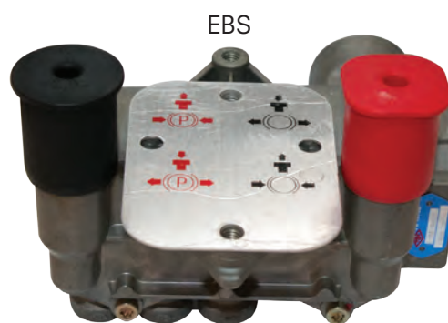
PARK RELEASE EMERGENCY VALVE КЛАПАН АВАРИЙНОГО РАСТОРМАЖИВАНИЯ
